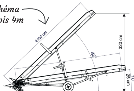
Schéma tapis 5m
