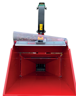
Vue de face : Trémie large 72x55 cm
